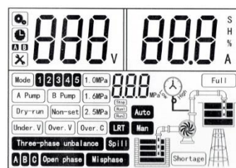
Diagrama de visualización de la pantalla LCD
