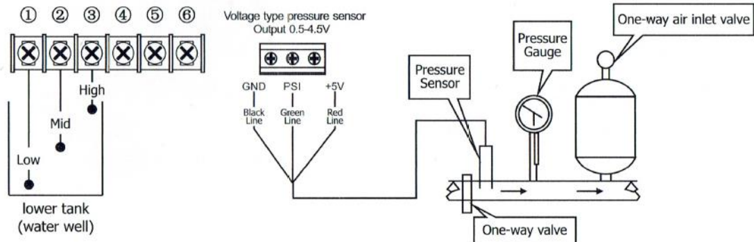
Diagrama de instalación de presión en cañería
