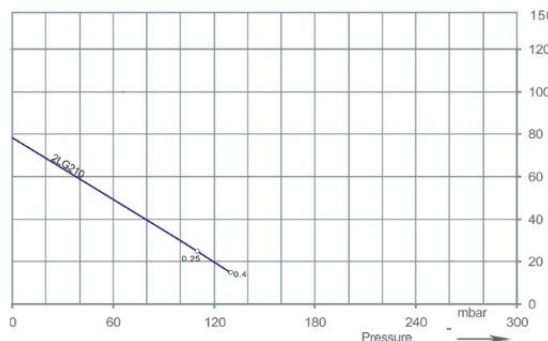
Gráfico de selección del compresor 50 HZ
