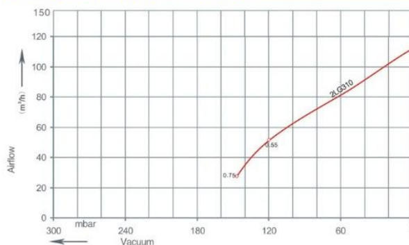
Gráfico de selección del compresor 50 HZ
