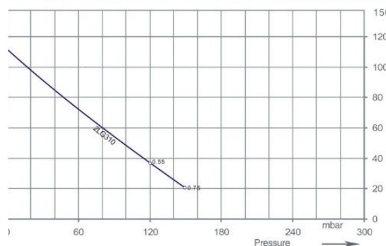
Gráfico de selección del compresor 50 HZ
