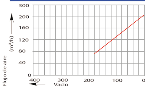
Gráfico de selección de vacío 50 HZ
