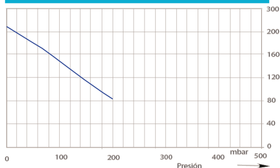
Gráfico de selección del compresor 50 HZ
