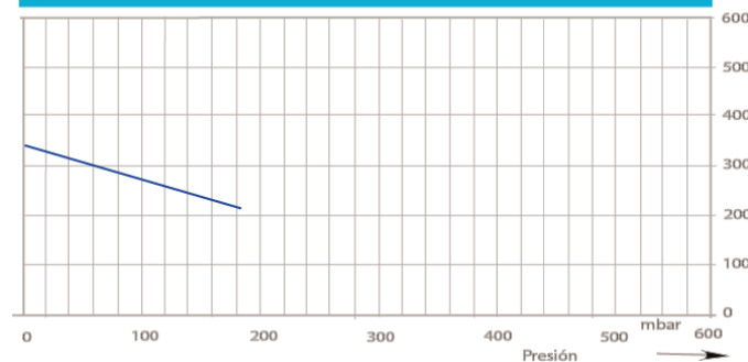
Gráfico de selección del compresor 50 HZ
