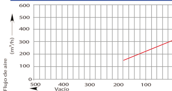
Gráfico de selección del compresor 50 HZ
