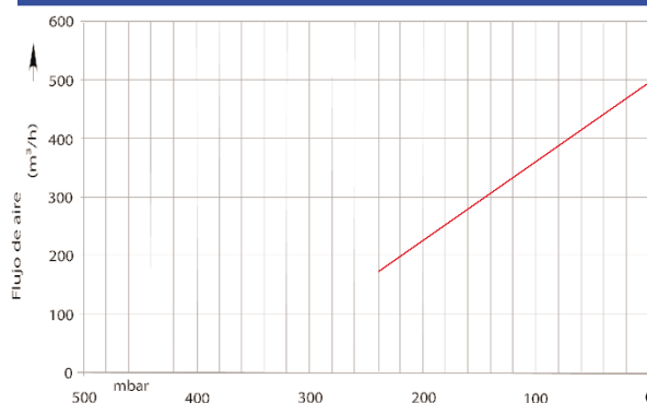
Gráfico de selección del compresor 50 HZ
