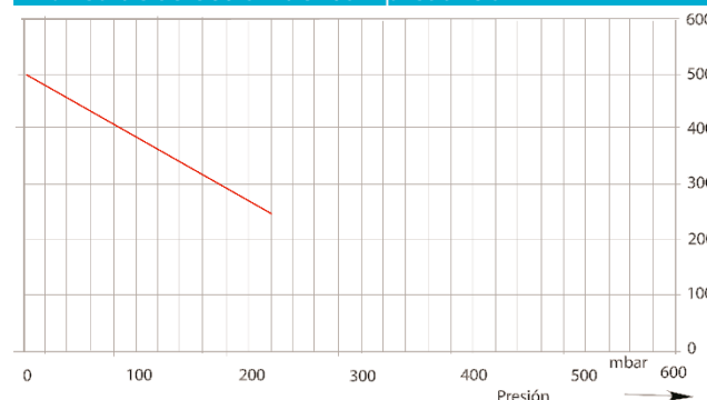
Gráfico de selección del compresor 50 HZ
