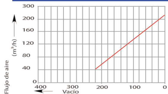
Gráfico de selección del compresor 50 HZ
