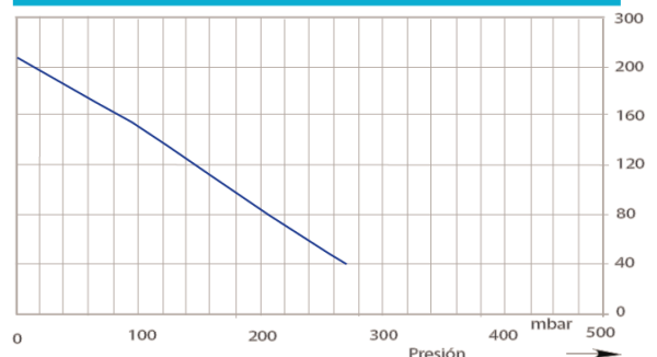
Gráfico de selección del compresor 50 HZ
