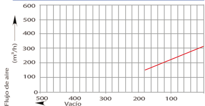
Gráfico de selección del compresor 50 HZ
