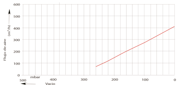
Gráfico de selección del compresor 50 HZ
